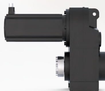
FLACHGETRIEBE: das Getriebe zum einfachen Anbau bis 8.900 Nm
