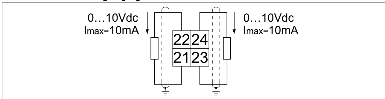
Abbildung 11: Beispiel zum Anschluss der Analogausgänge
