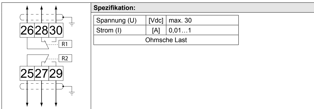
Abbildung 9: Beispiel zum Anschluss der Relaisausgänge
