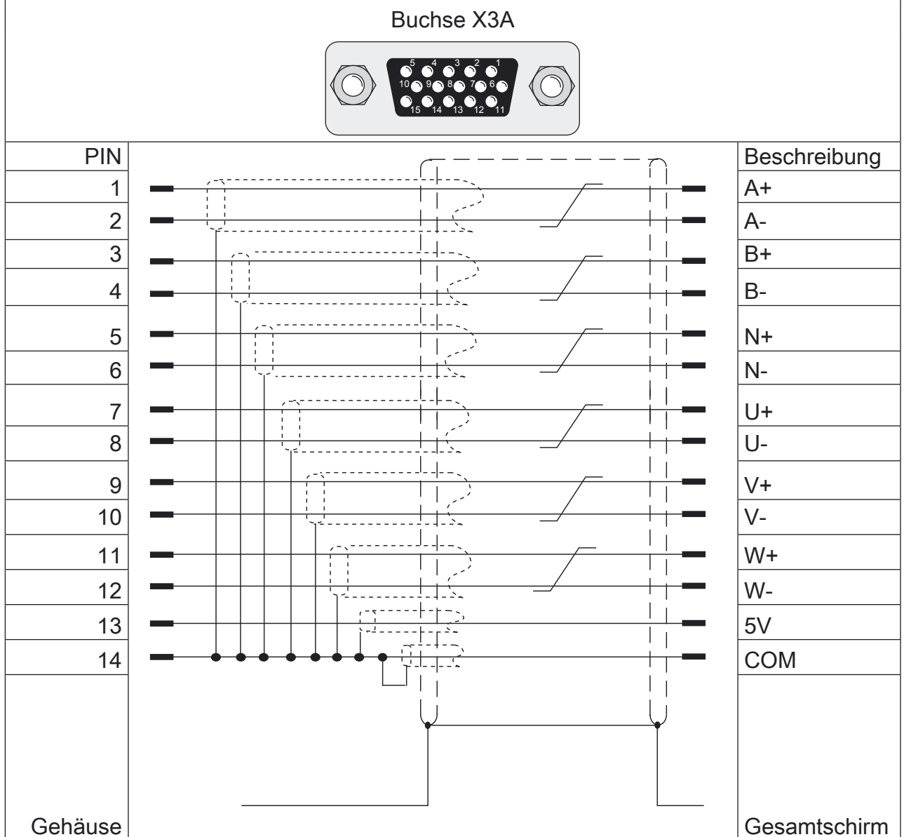
Bild 2.2.5 Anschluss des Gebers
