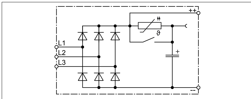
Abbildung 7: Eingangsbeschaltung/Antriebsstromrichtertyp
