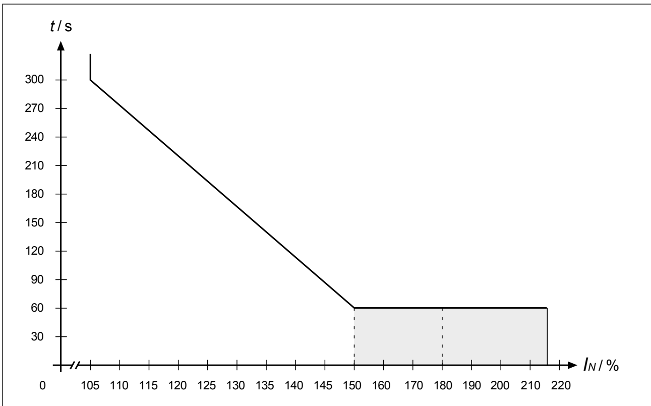
Abbildung 2: Überlastkennlinie
