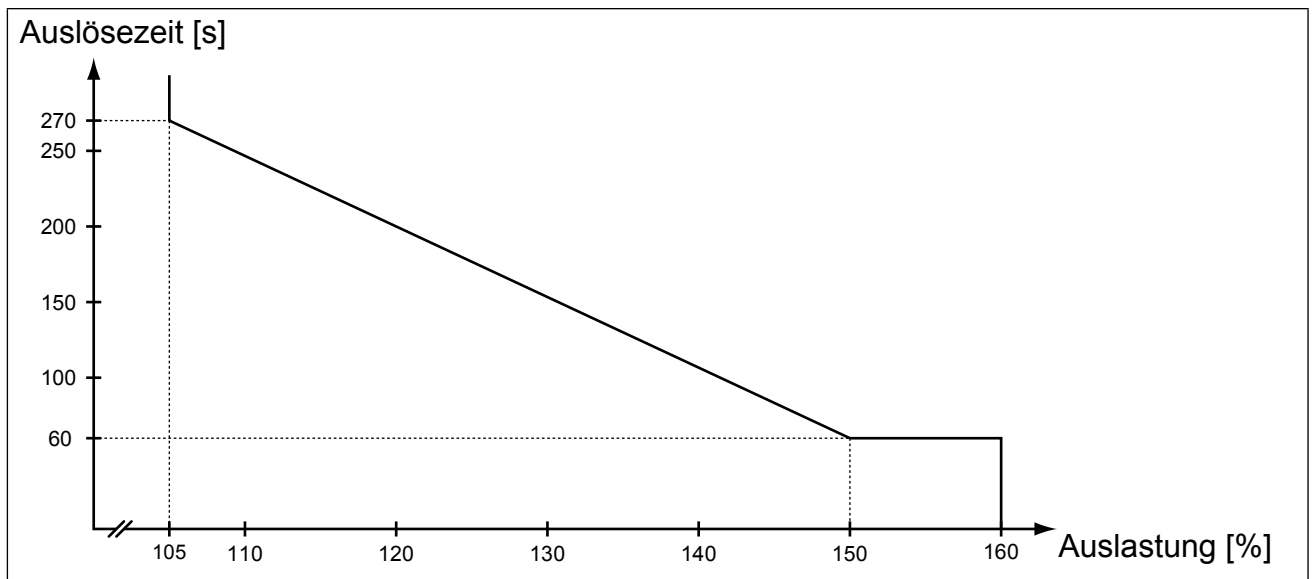
Abbildung 1: Überlast (OL)-Funktion
