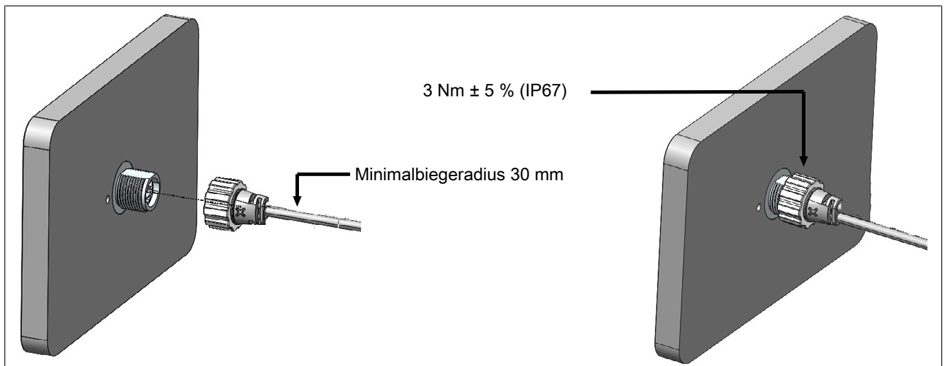
Abb. 1: Montage C6 X1-C1
