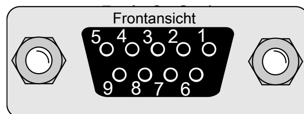
Abb. 19: X10 INTERBUS Eingang
