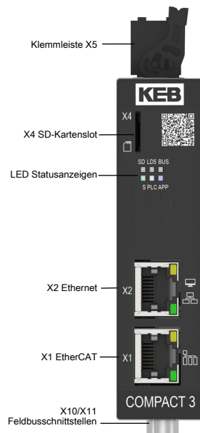
Abb. 3: C6 COMPACT 3 Frontansicht Modell 4
