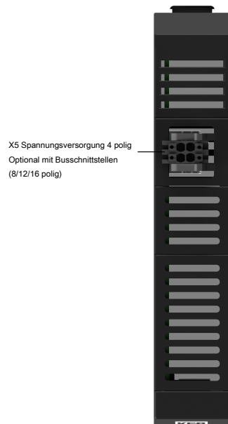
Abb. 4: C6 COMPACT 3 oben Modell 1 und 2
