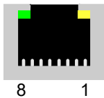
Abb. 17: Buchse RJ45 Frontansicht
