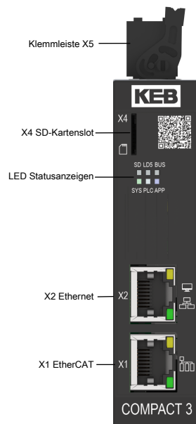
Abb. 1: C6 COMPACT 3 Frontansicht Modell 1 und 3
