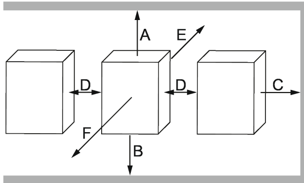
Abb. 12: Einbauabstände
