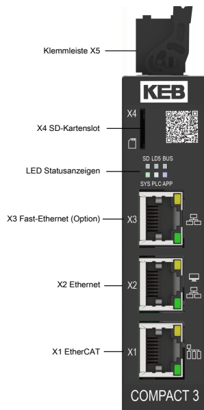
Abb. 2: C6 COMPACT 3 Frontansicht Modell 2
