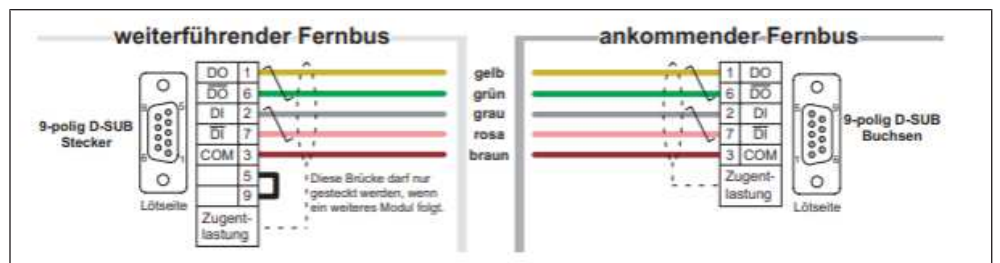
Abb. 21: Belegung INTERBUS-Fernbuskabel
