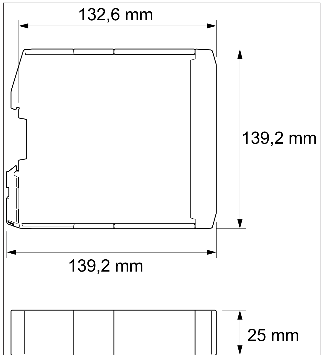
Abb. 11: Abmessungen COMPACT 3
