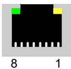
Abb. 15: Buchse RJ45 Frontansicht
