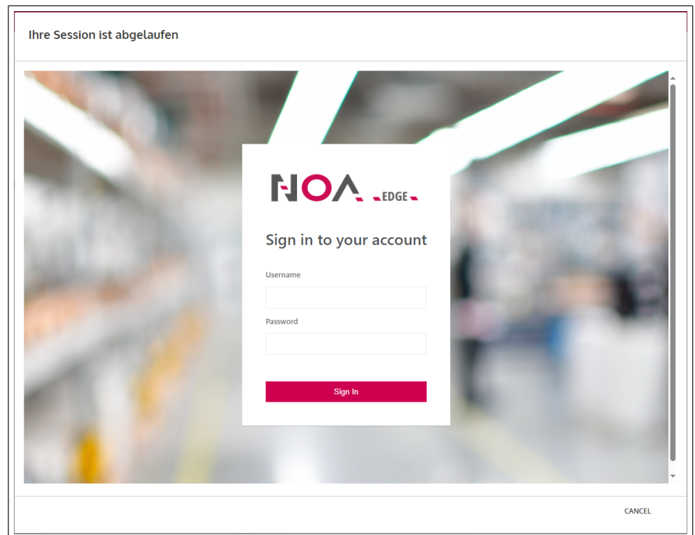
Abb. 26: Automatischer Logout
