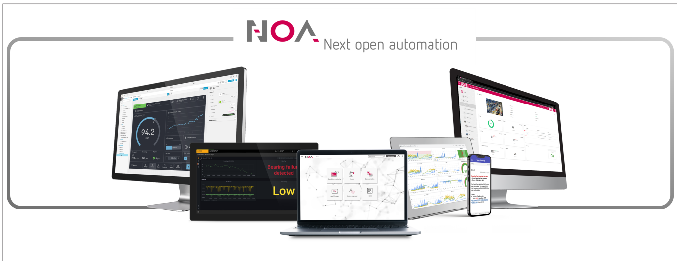
Abb. 39: NOA Portal
