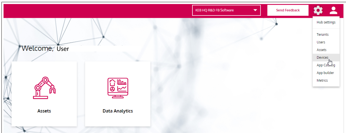
Abb. 40: Geräteliste aufrufen
