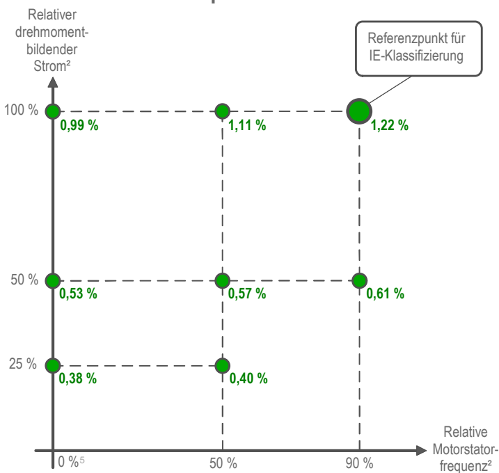
Relative Verluste in den Arbeitspunkten
