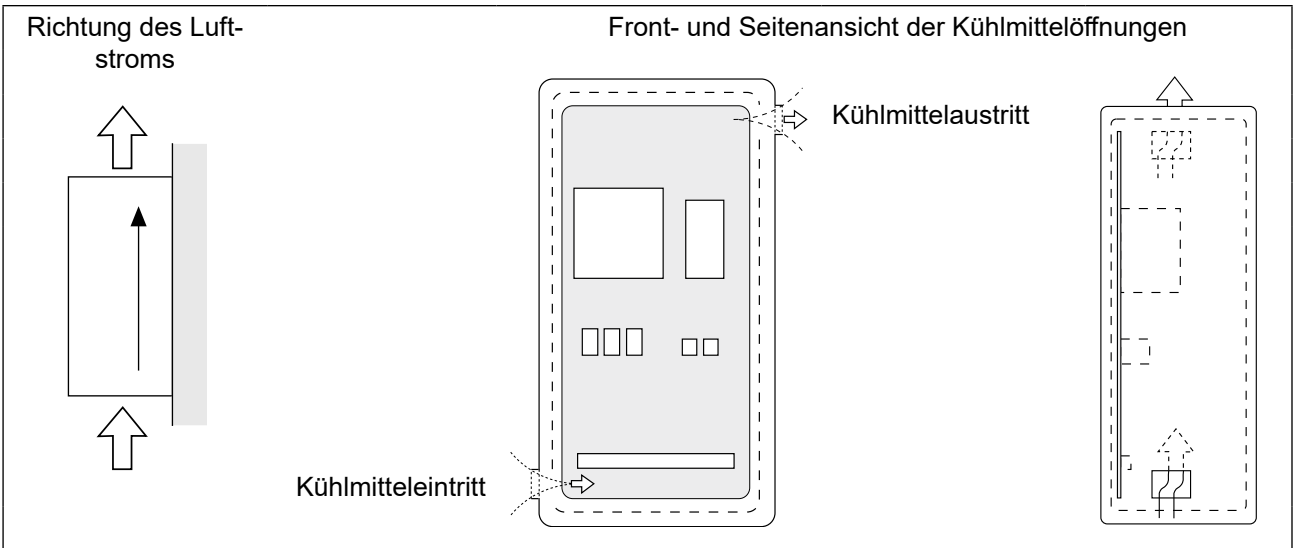
Abbildung 15: Schaltschranklüftung
