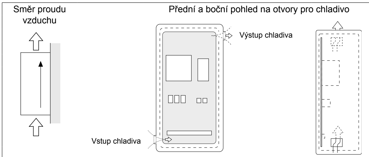
Ilustrační 5: Ventilace rozvaděče
