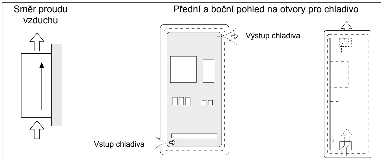
Ilustrační 6: Ventilace rozvaděče
