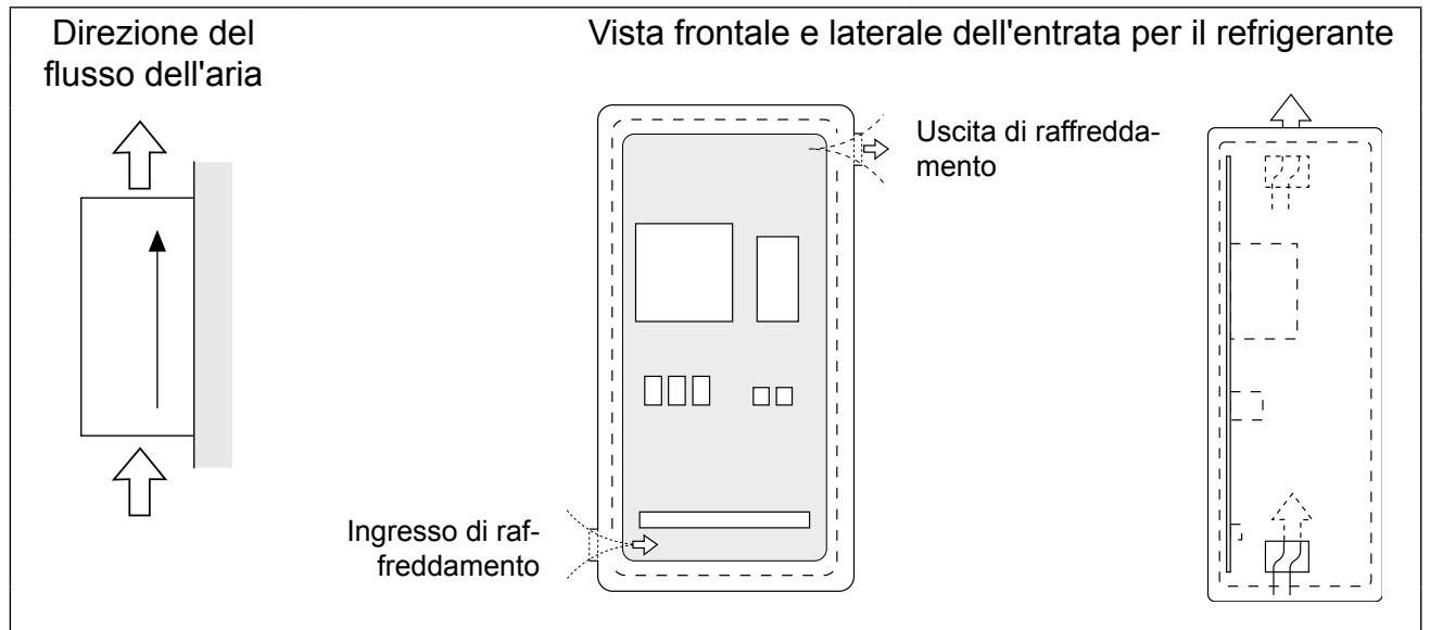
Figura 5: Ventilazione del quadro elettrico
