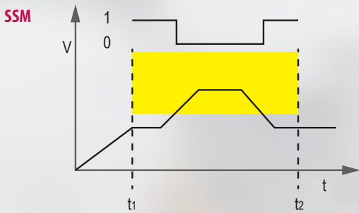
安全速度监控(f=0 Hz)
