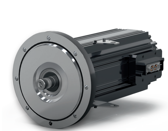
6 MW 变桨电机
