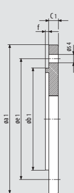
Bride B5 (1)
